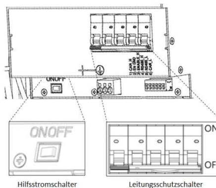
Bild 1: LG RESU Hochvoltbatteriespeicher – Trennvorrichtungen, Sicherungshebel und Hilfsschalter
