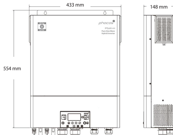
PSW-H-5KW-120/48V
