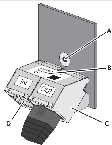
Abbildung 1: Aufbau der SI-COMSMA.BG1
