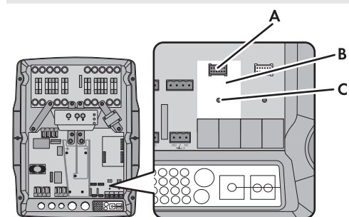
Abbildung 2: Einbauort und Anschluss der SI-COMSMA.BG1
