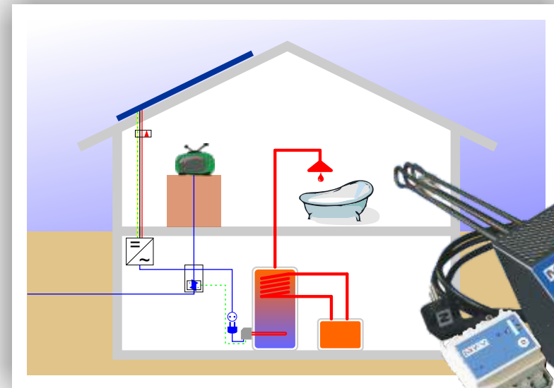
AC ELWA
